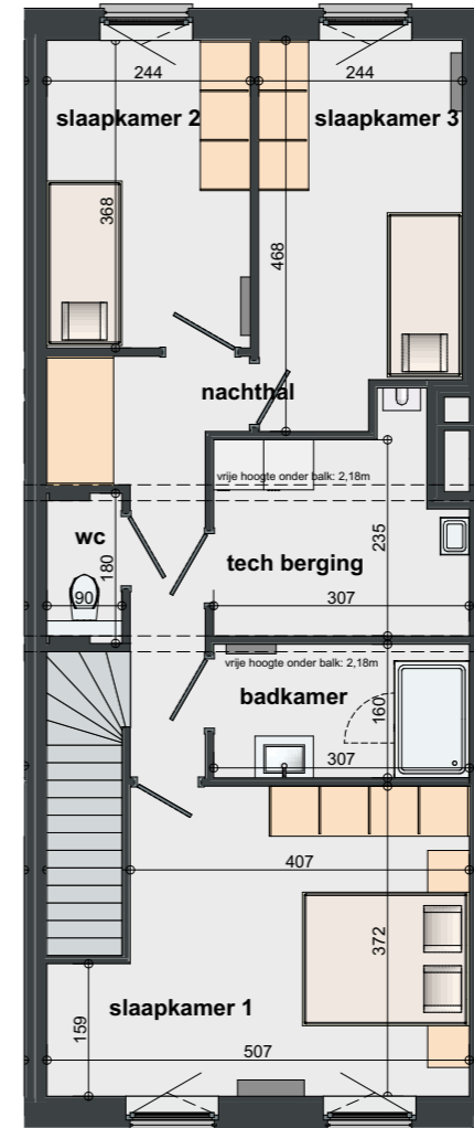
1e verdieping 1:100
