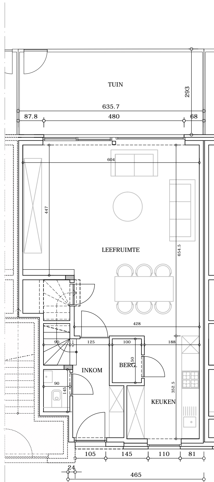
GELIJKVLOERS
