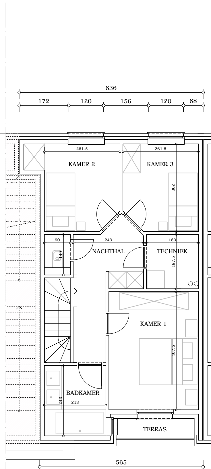
VERDIEPING 1
