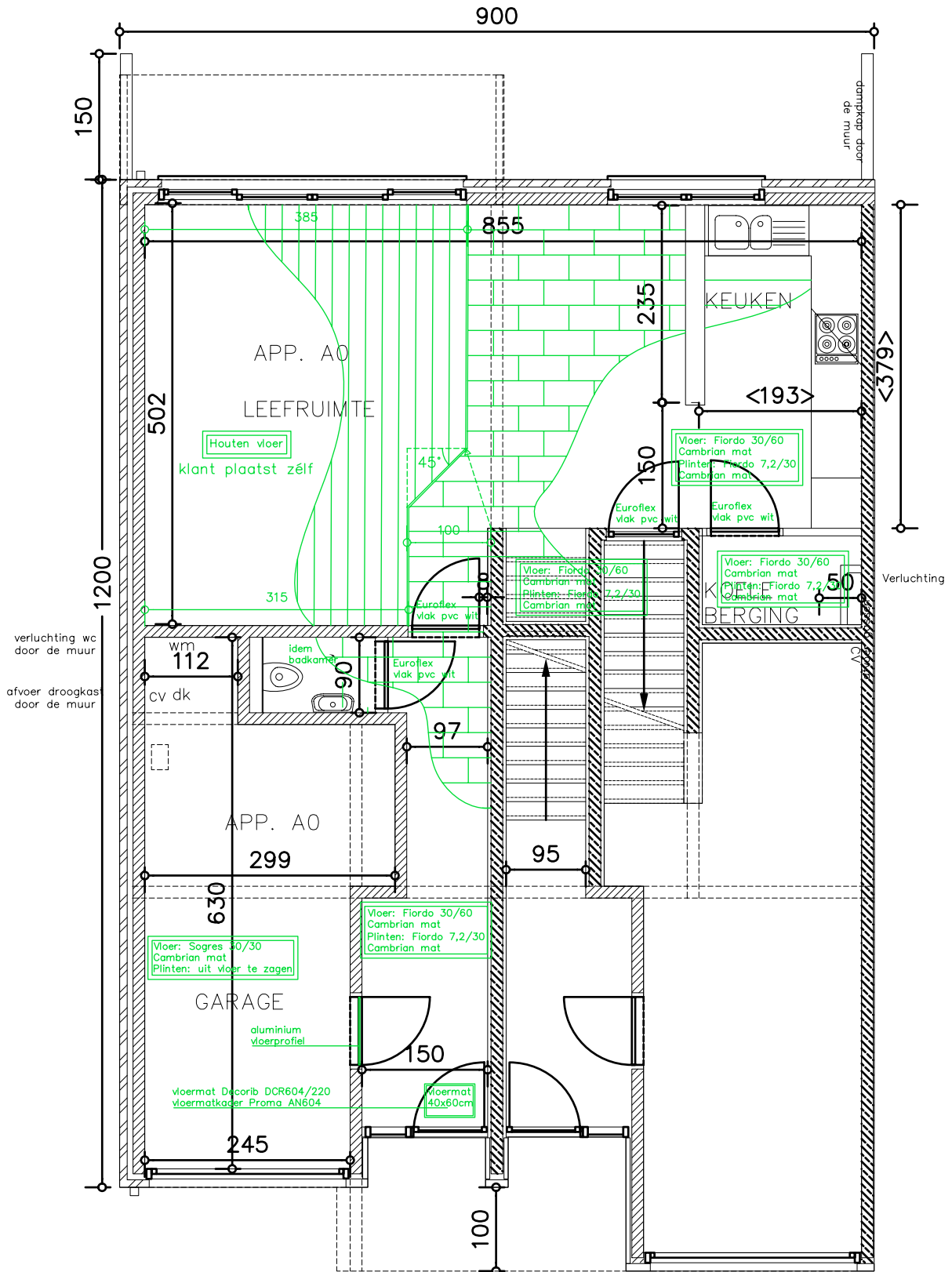
GRONDPLAN
