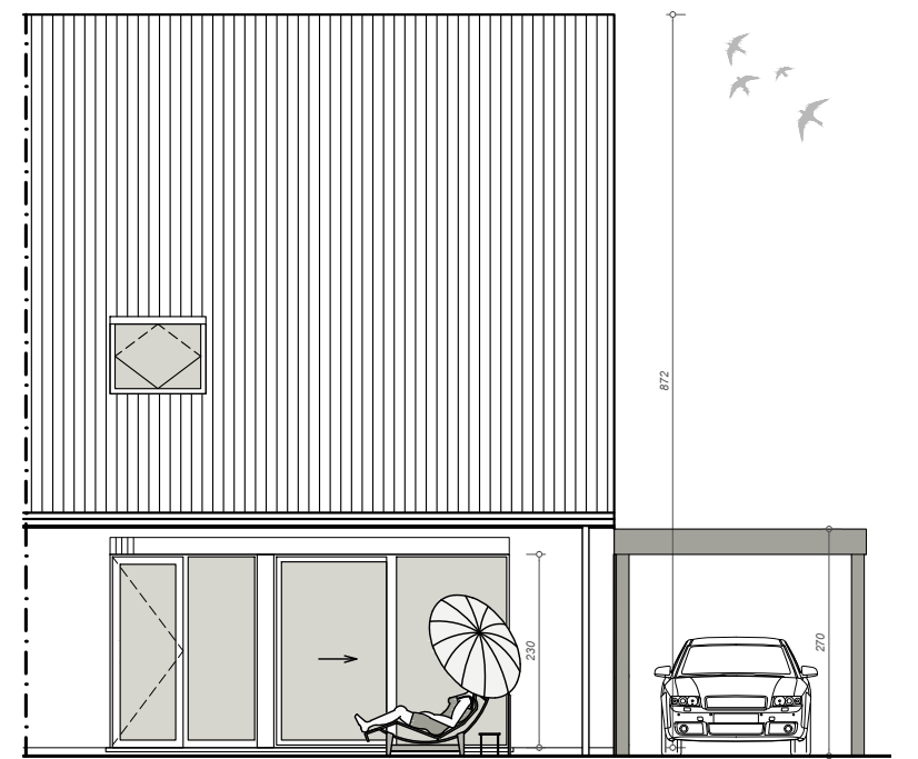
ACHTERGEVEL
