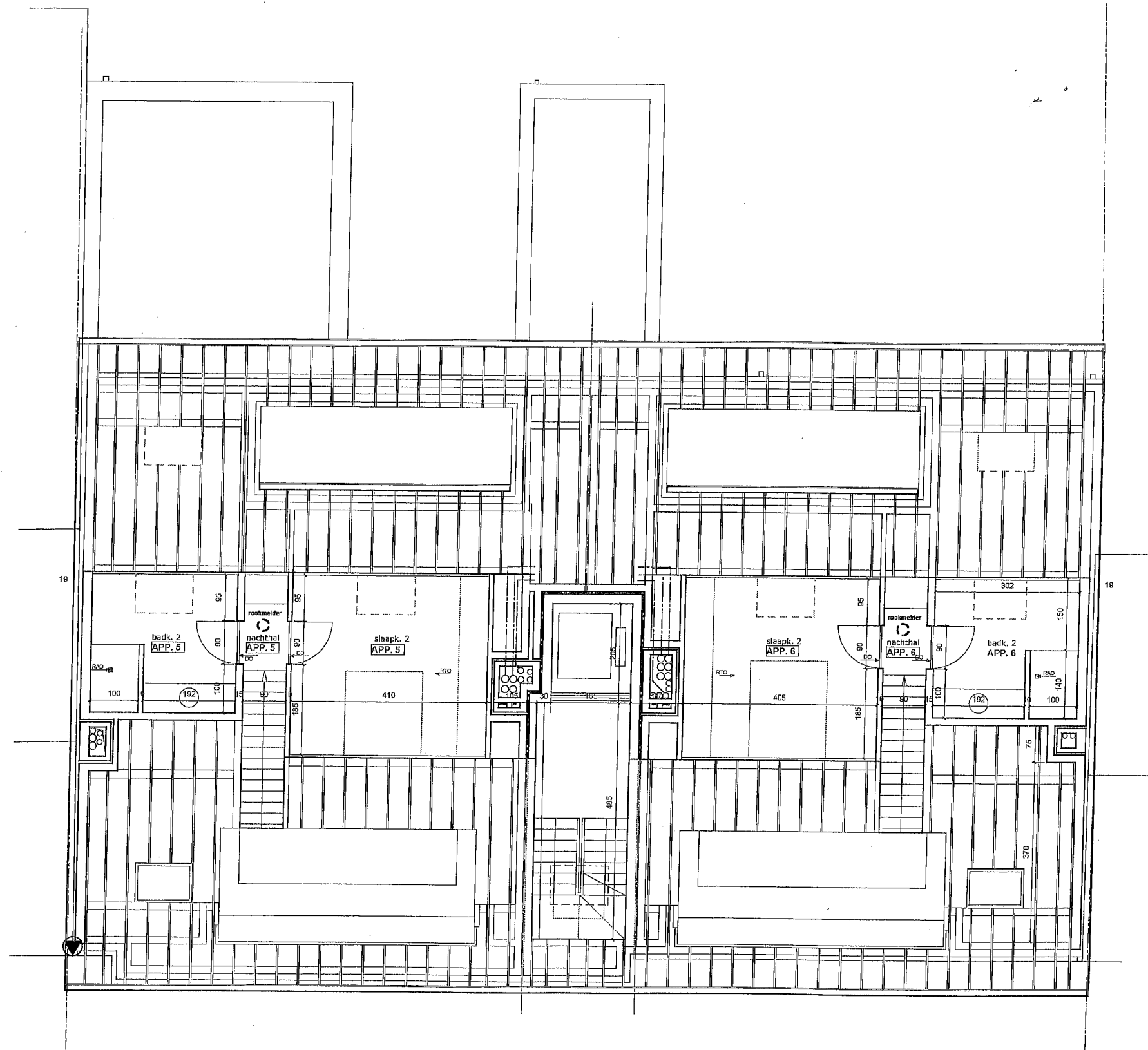
appartementengebouw nieuwe toestand dakverdieping - duplex
