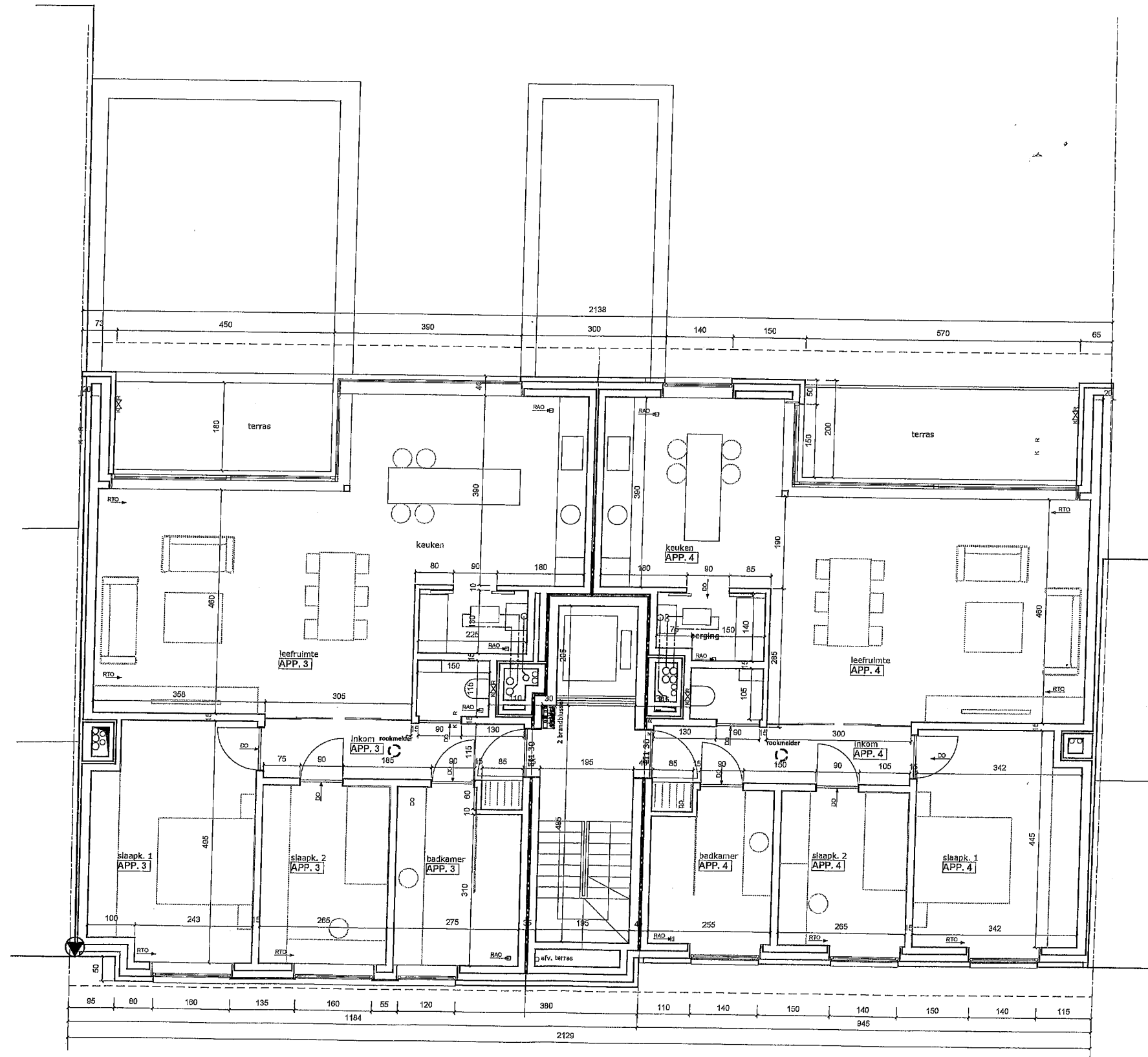
appartementengebouw nieuwe toestand verdiepingsplan 1
