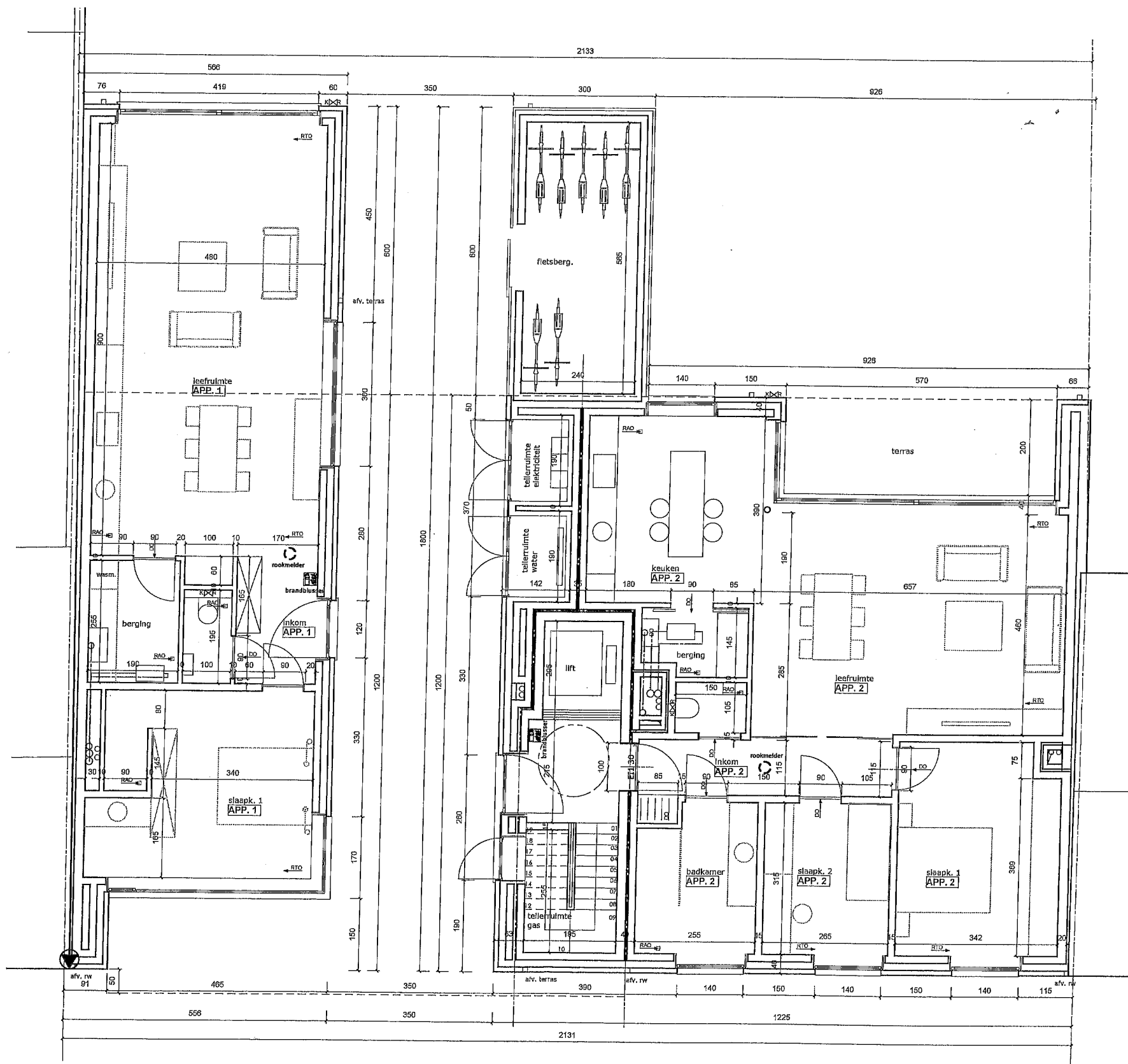
appartementengebouw nieuwe toestand gelijkvloersplan
