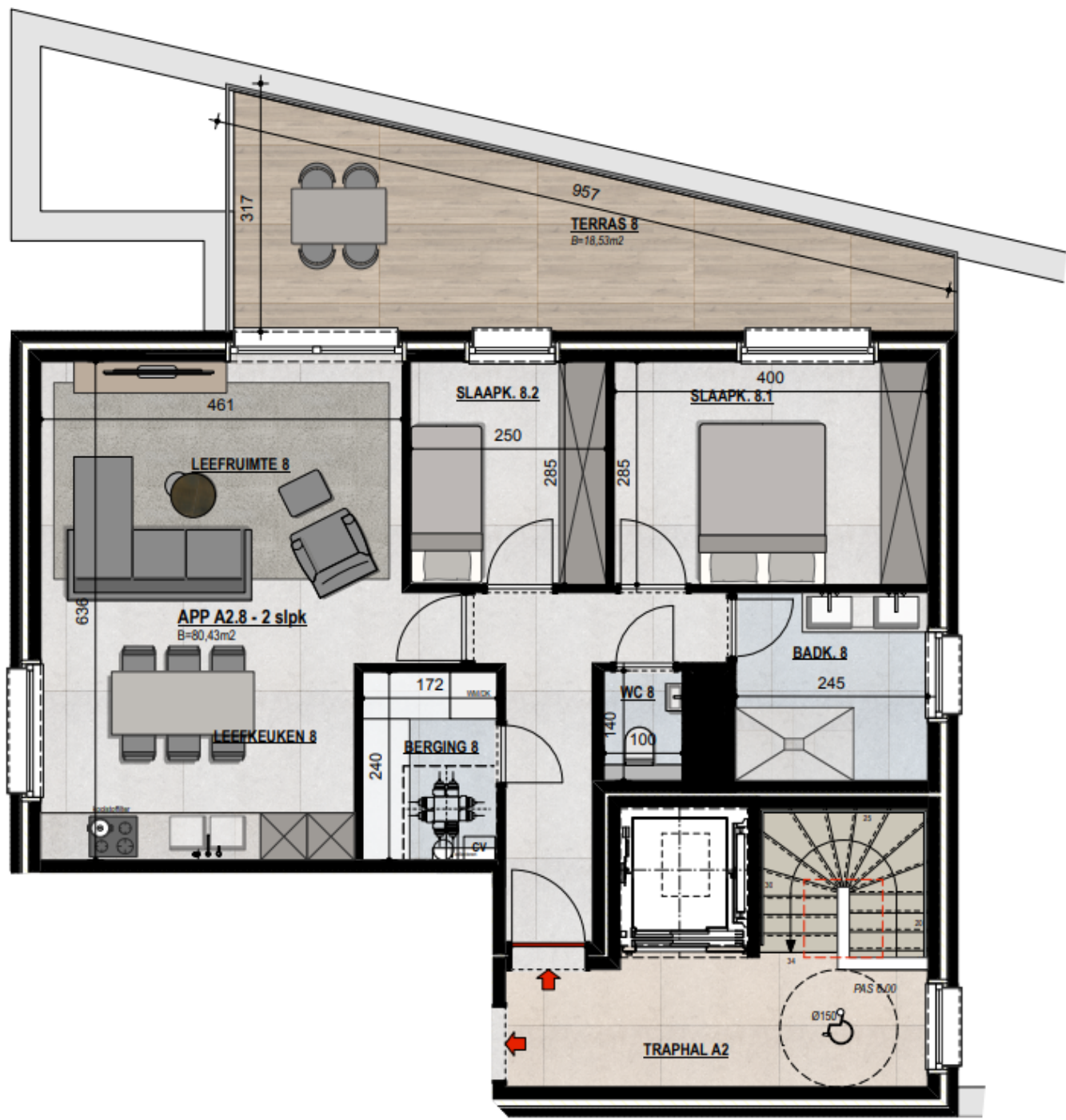
GRONDPLAN - 2de VERDIEPING - APP A2.8 - 80,43 m2
