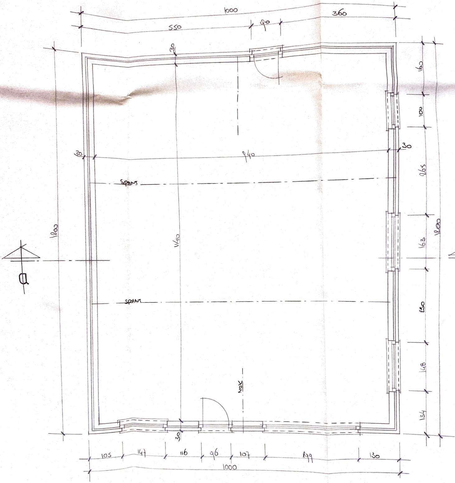
grondplan
