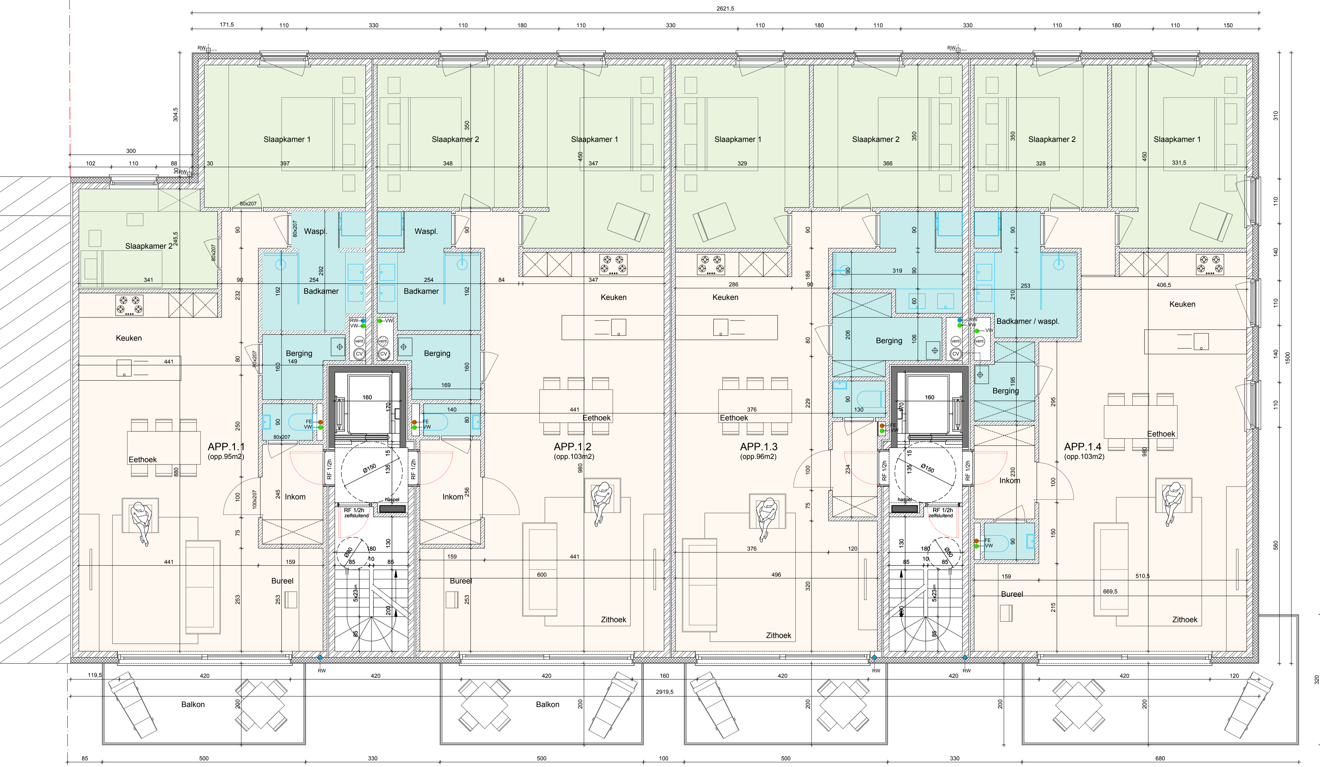
- VERDIEPING +1° -
