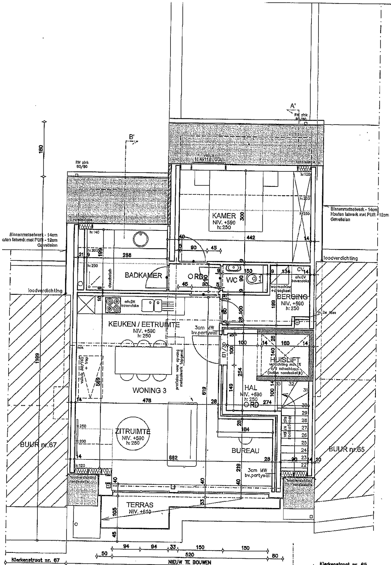
VERDIEPING 2 Renterlepel 000 = L.12.00 H deurtintelen = 207cm (tenzij anders vermeld op plan) 0 1 2 3 4 5m
