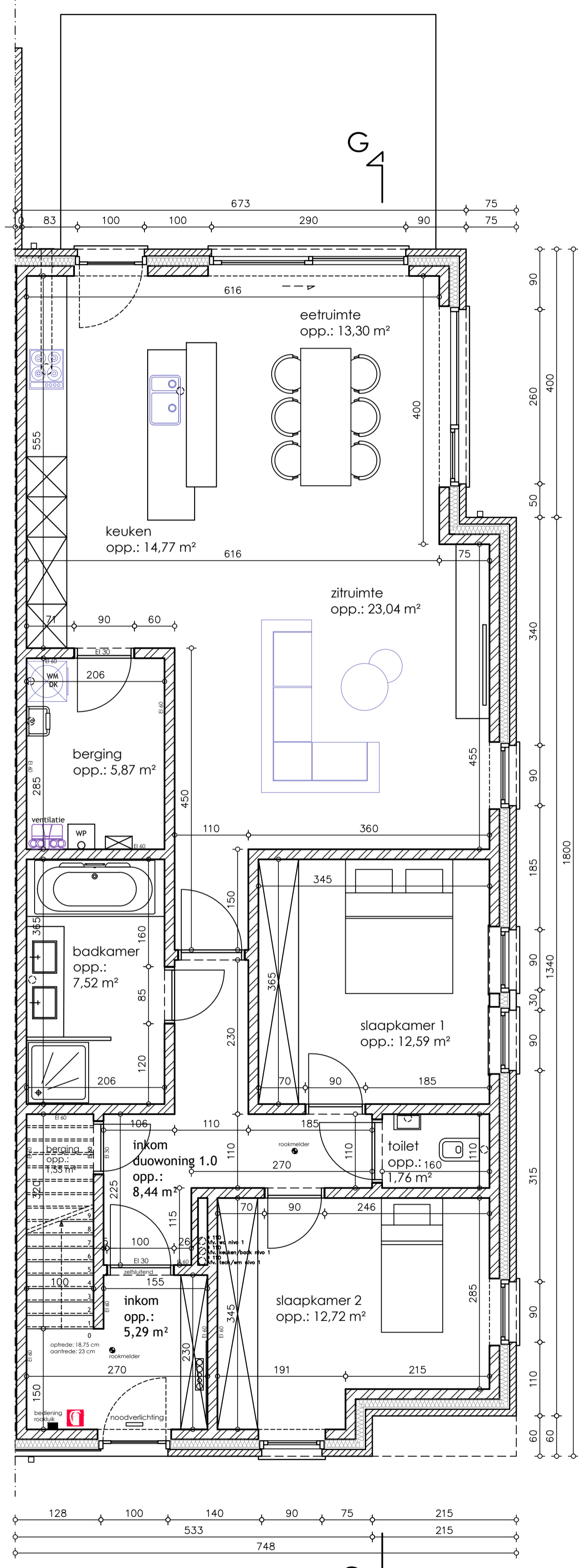
GRONDPLAN: DUO-WONING 1 SCHAAL 1:50
