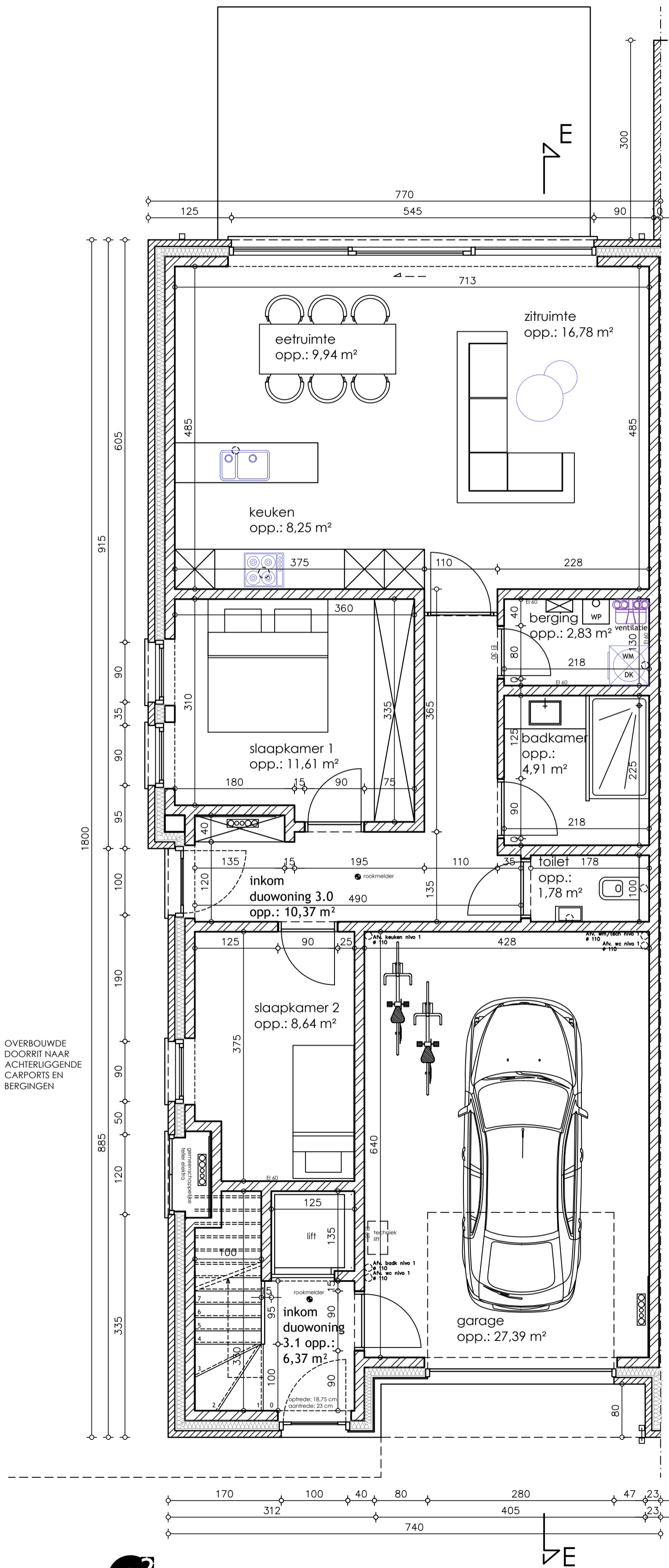
GRONDPLAN: DUO-WONING 3 SCHAAL 1:50
