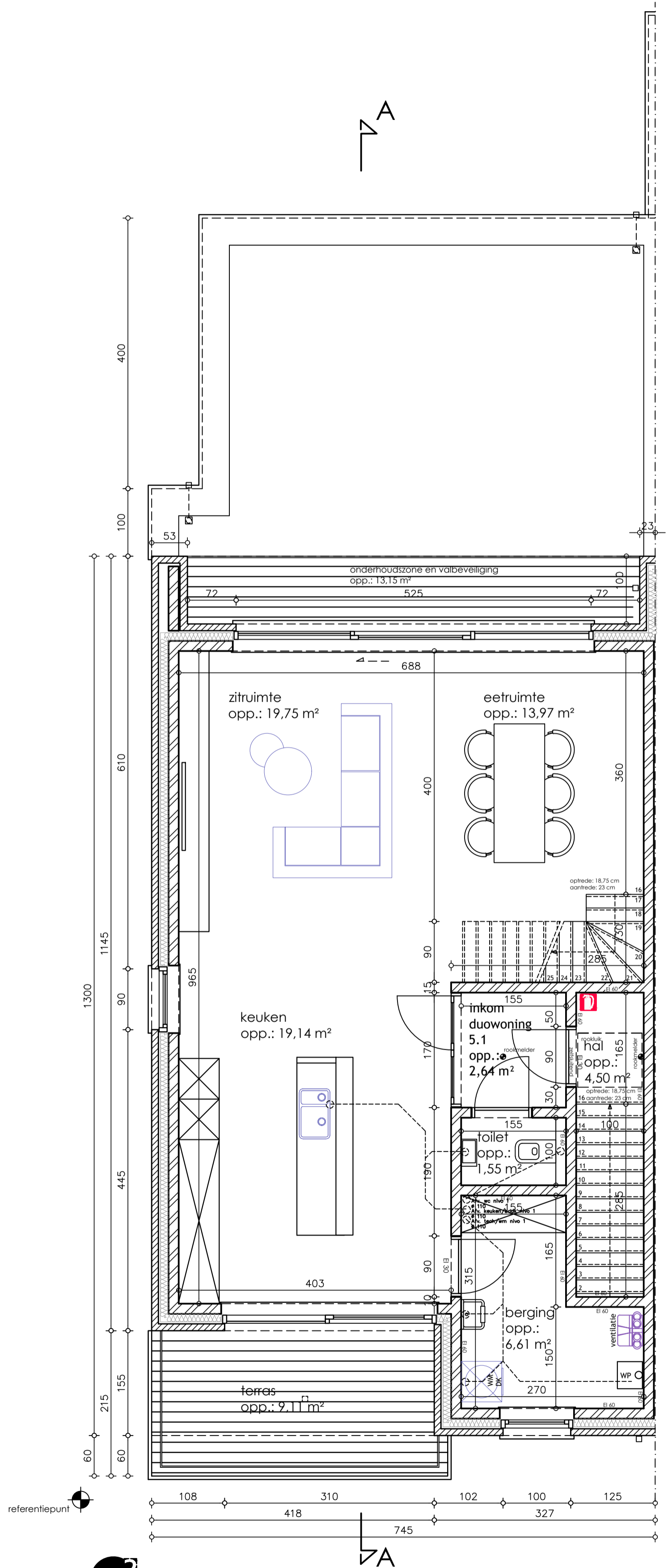
A 2 A-KWADRAAT architecten VERDIEPING 1: DUO-WONING 5 SCHAAL 1:50
