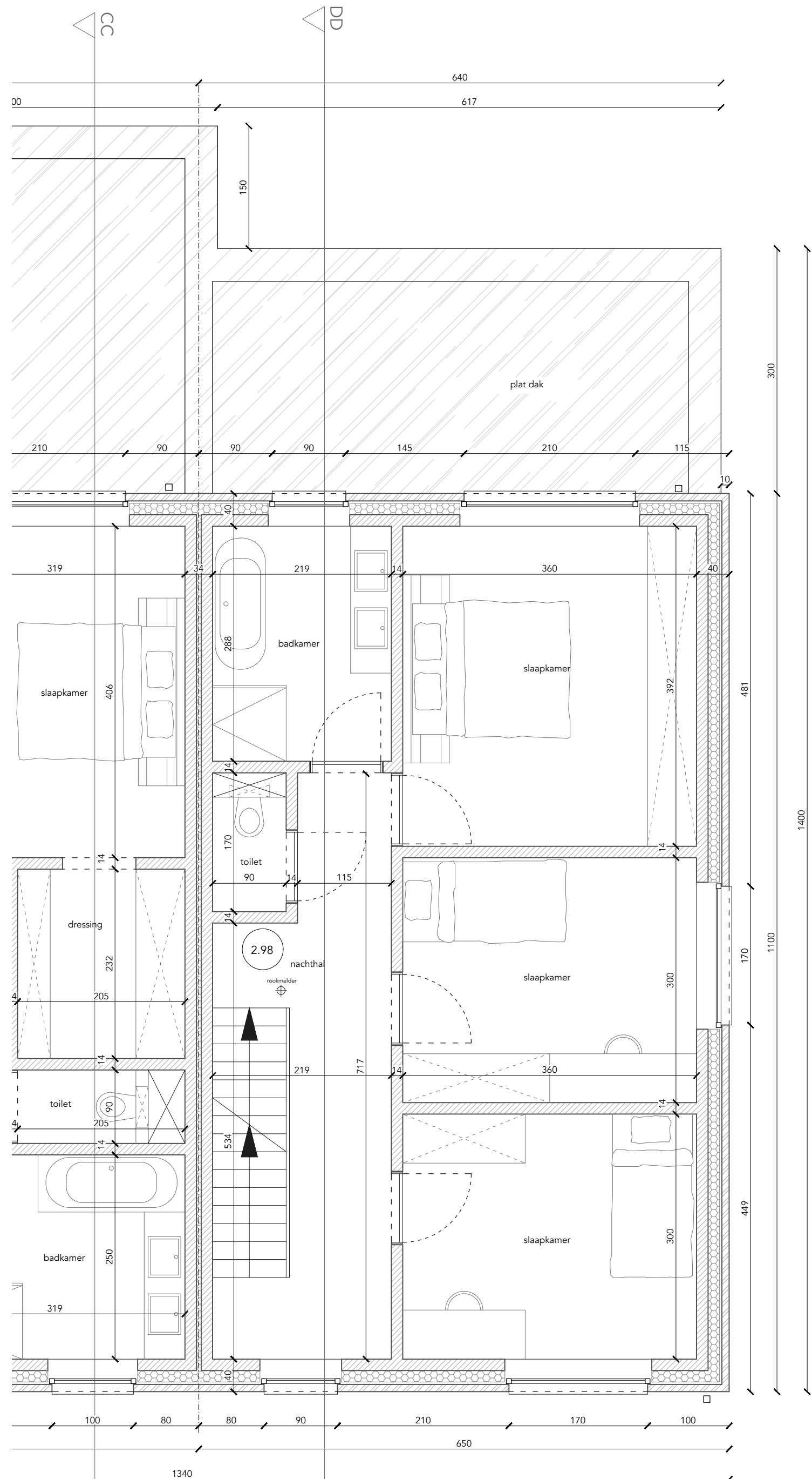
PLAN VERDIEPING (schaal 1/50)
