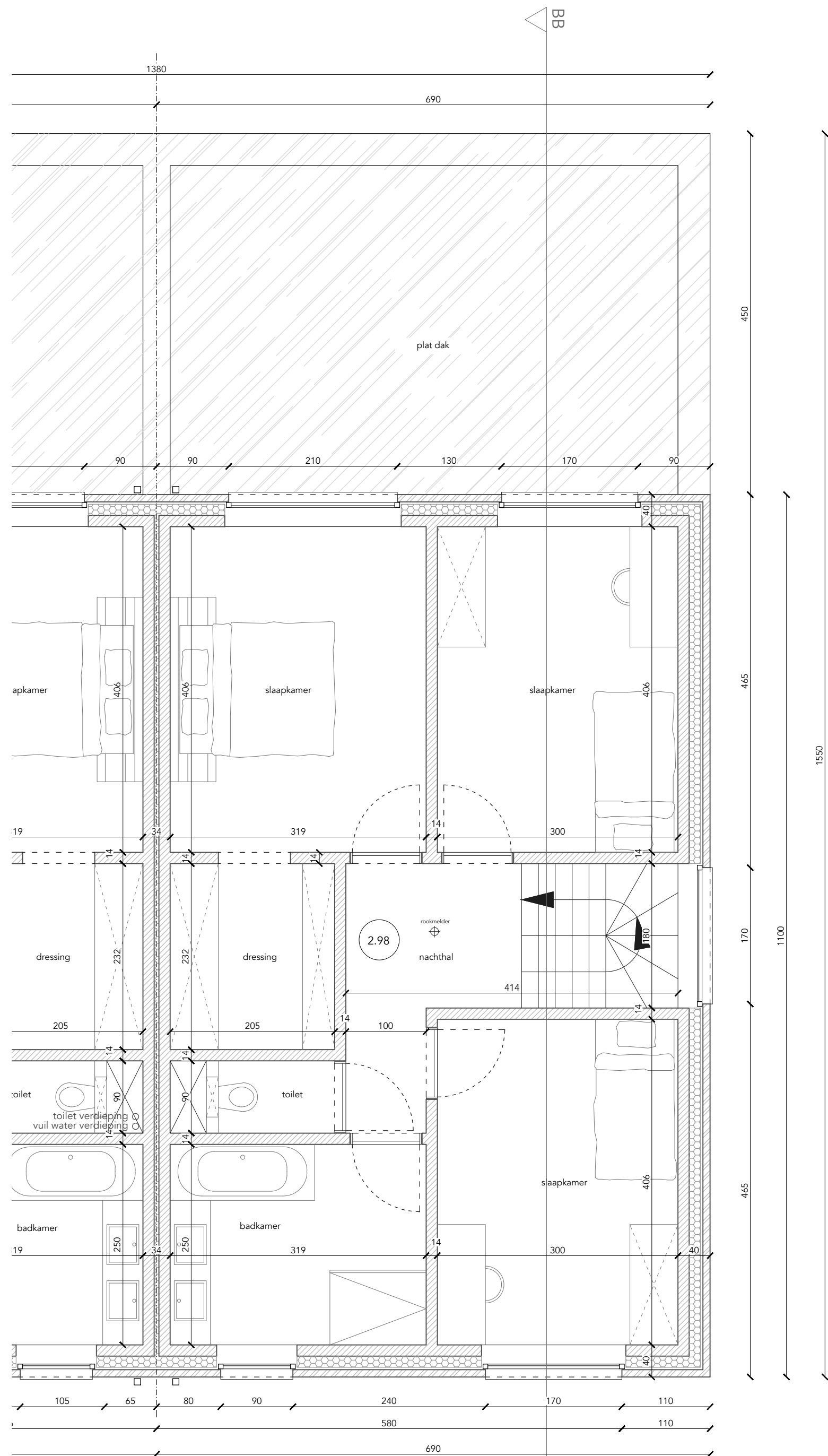
PLAN VERDIEPING (schaal 1/50)
