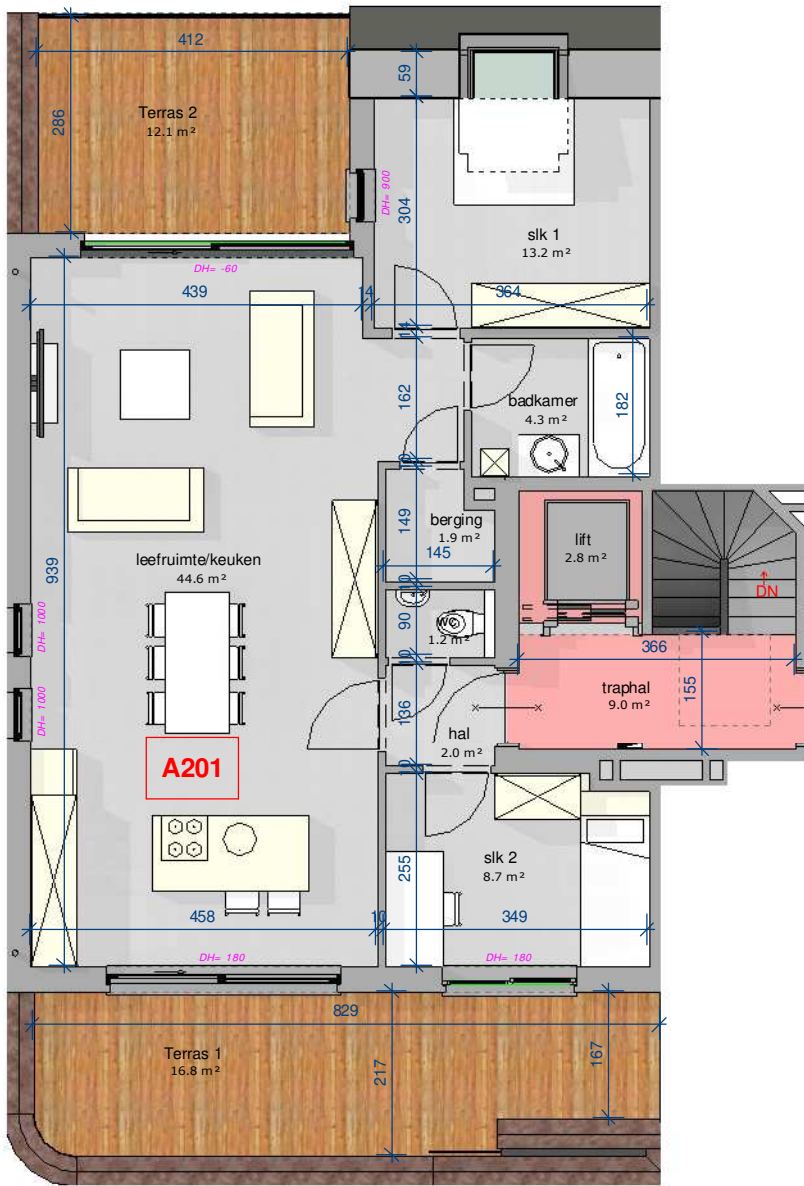
Niveau 2 - A201
