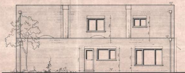
ACHTERGEVEL
