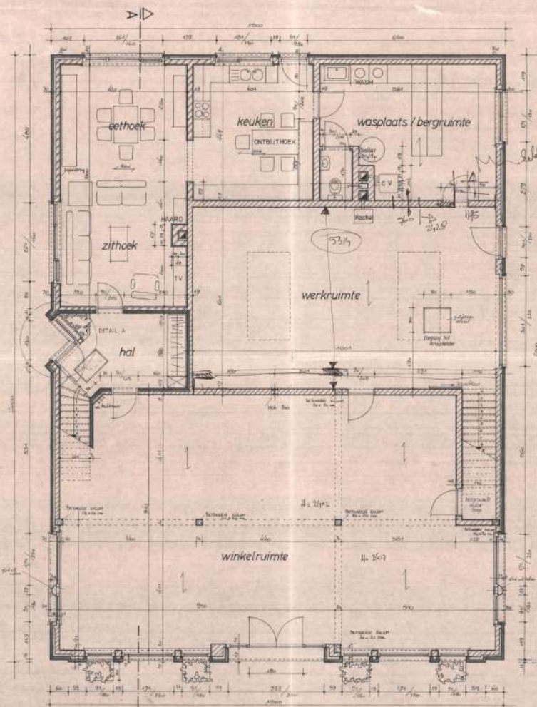
GELIJKVLOERS
