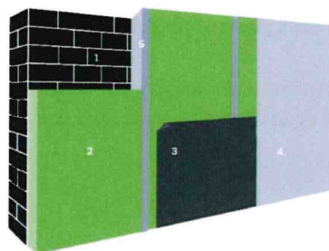
1. Buitengevel | 2. Isolatie | 3. Dampschermbekleding | 4. Binnenafwerking | 5. Stijl- en regelwerk (optioneel)
