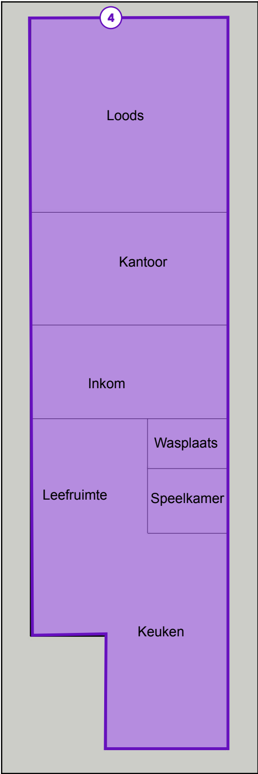
Legende van plan 1.4: Grondplan gelijkvloers
