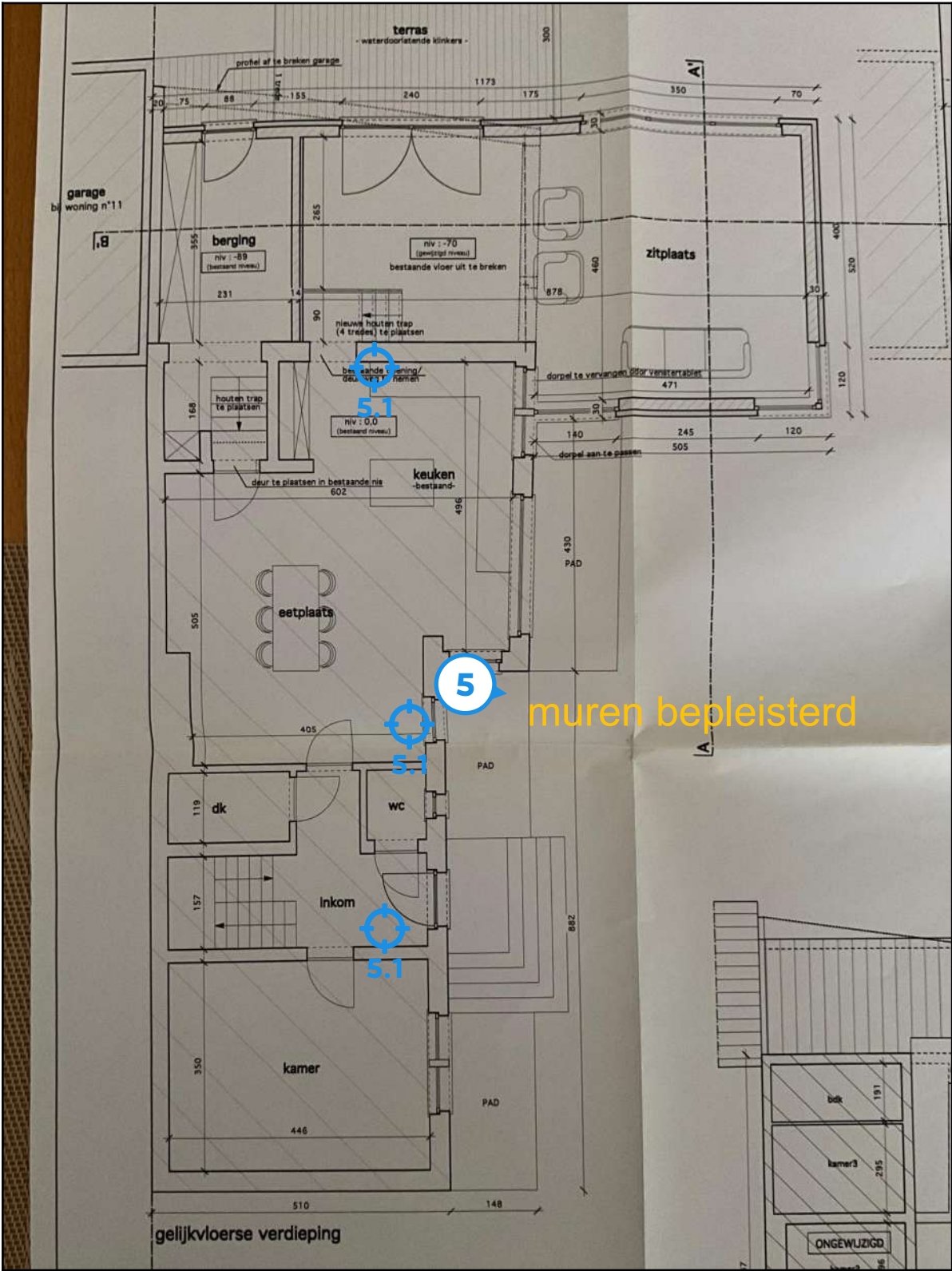
Legende van plan 1.2: Plan gelijkvloers wanden
