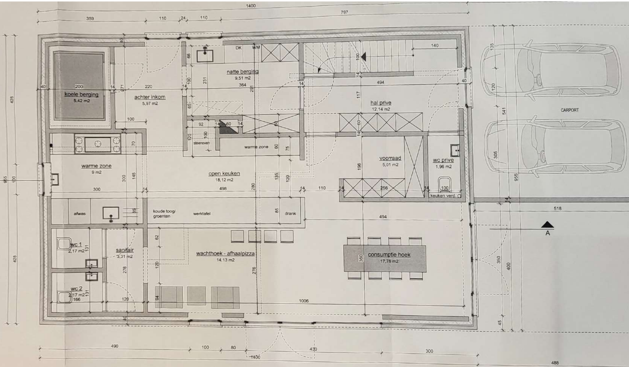
GRONDPLAN
