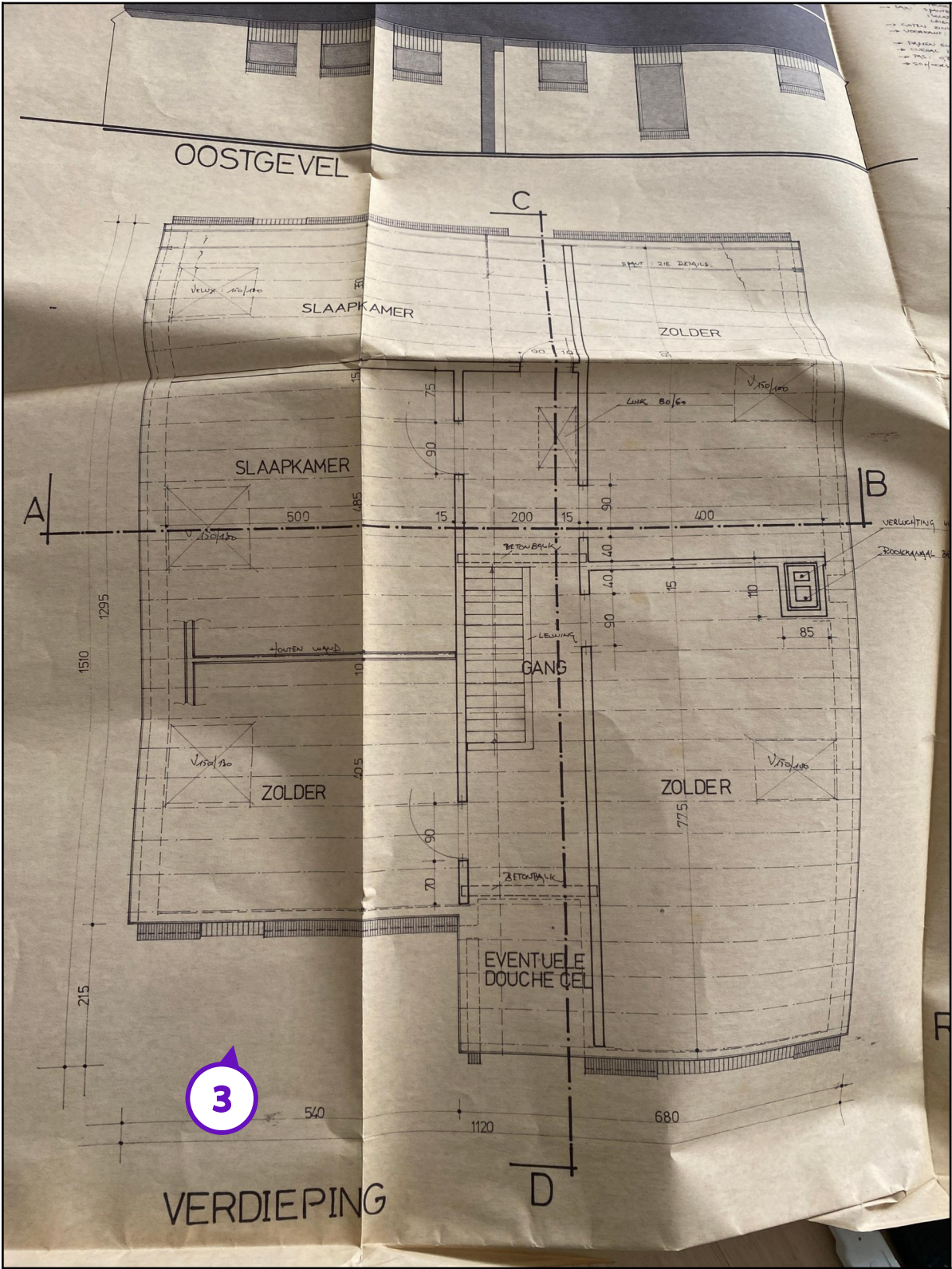
Legende van plan 1.2: 1e verdiep
