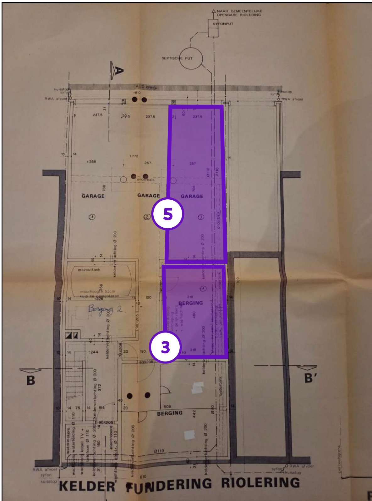
Legende van plan 1.6: Grondplan kelder+garage
