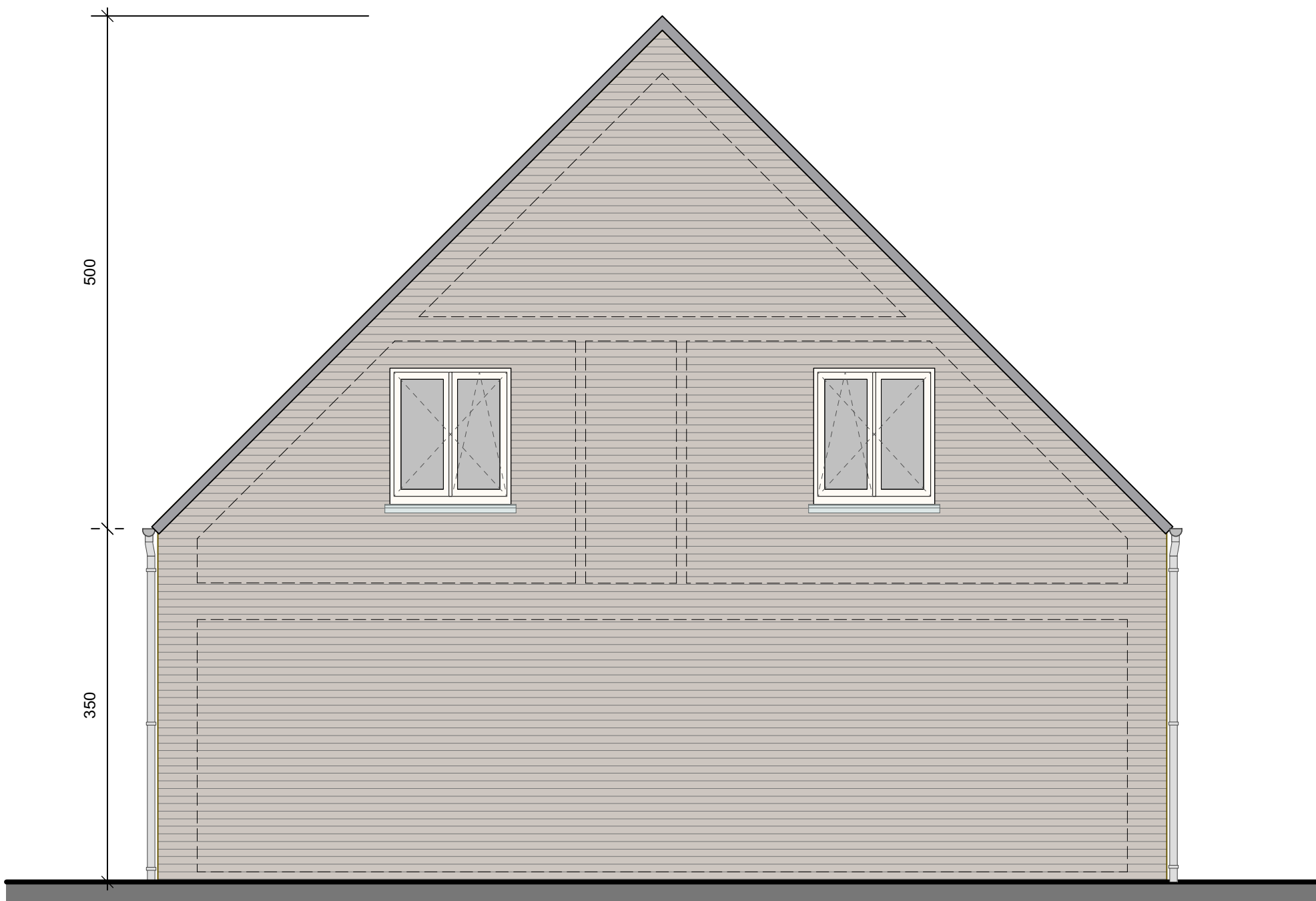
Zijgevel links
