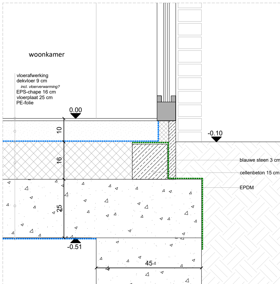
Detail B: principe raamaanzet
