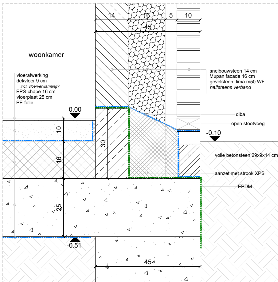
Detail A: principe funderingsaanzet
