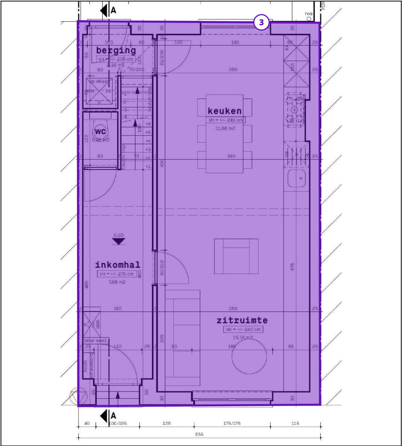
Legende van plan 1.6: Nieuw plan gelijkvloers
