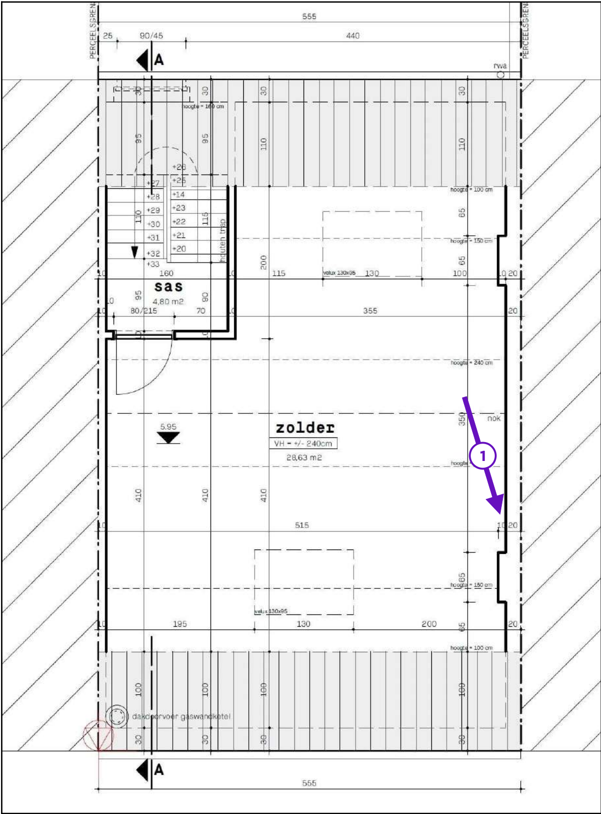
Legende van plan 1.10: Nieuw plan 2de
