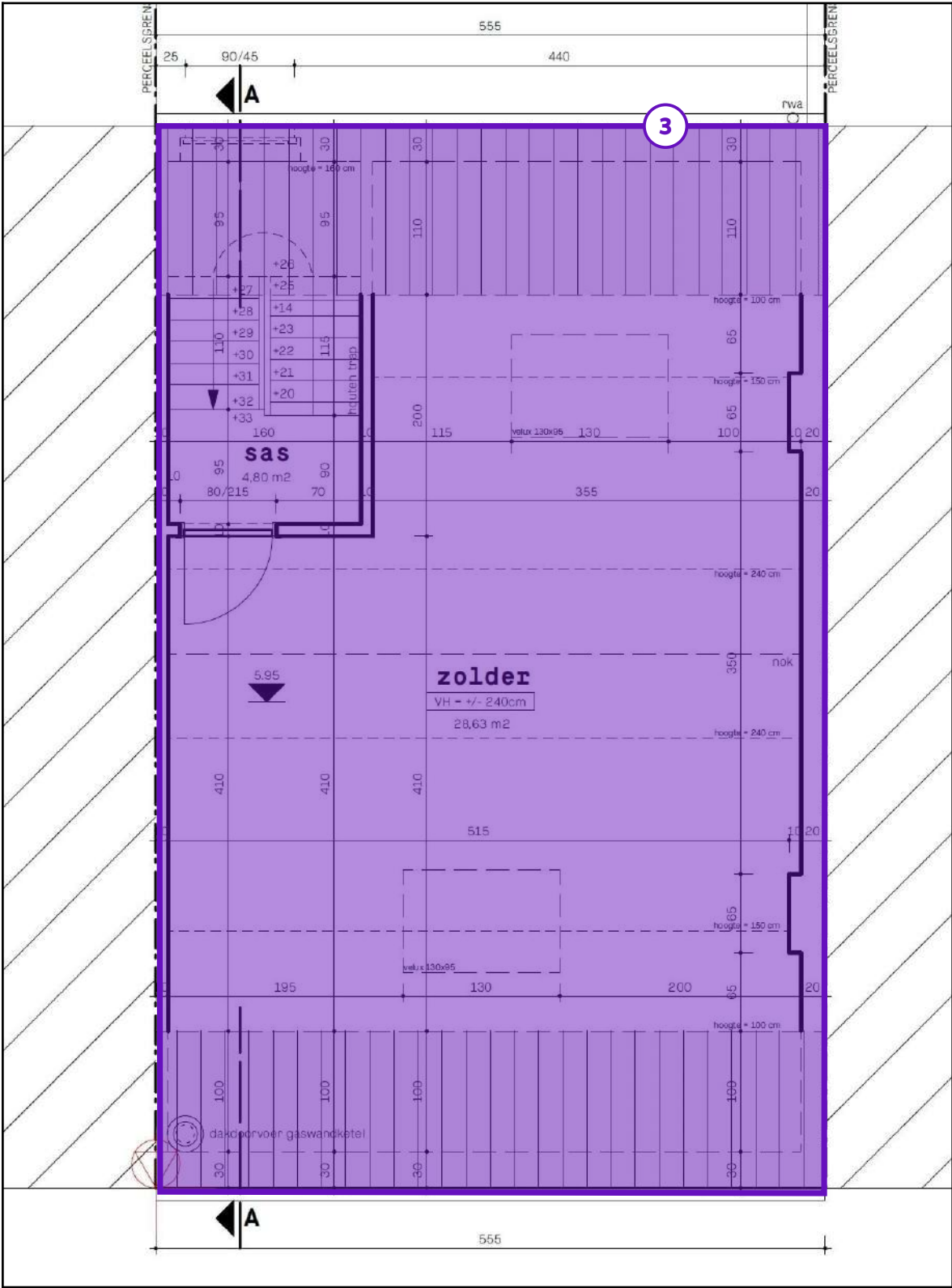
Legende van plan 1.8: Nieuw plan 2de
