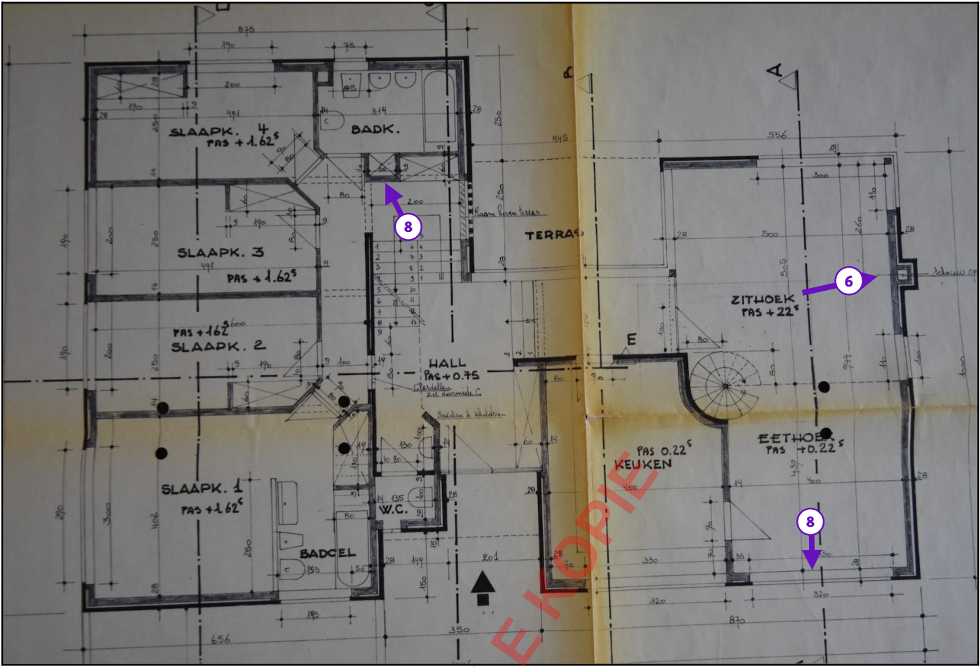
Legende van plan 1.6: Grondplan +0
