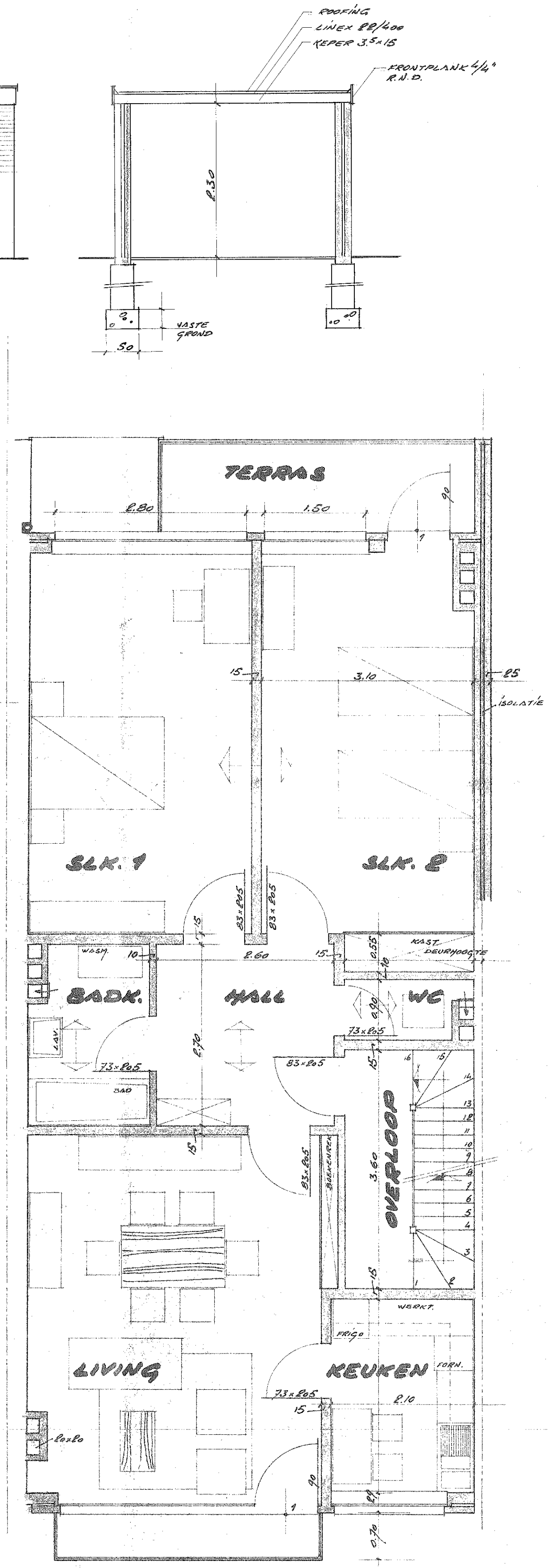
: 1e VERDIEPING
