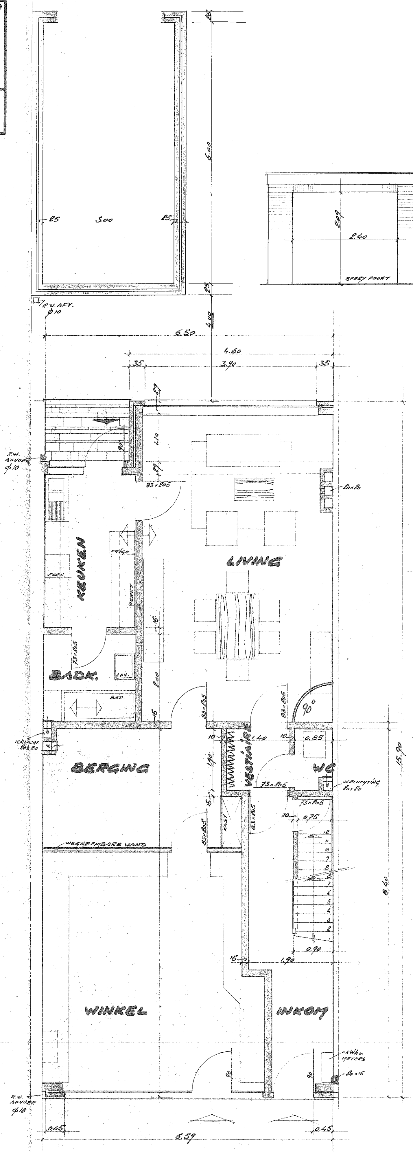
: GELUKVLOERS 1:50
