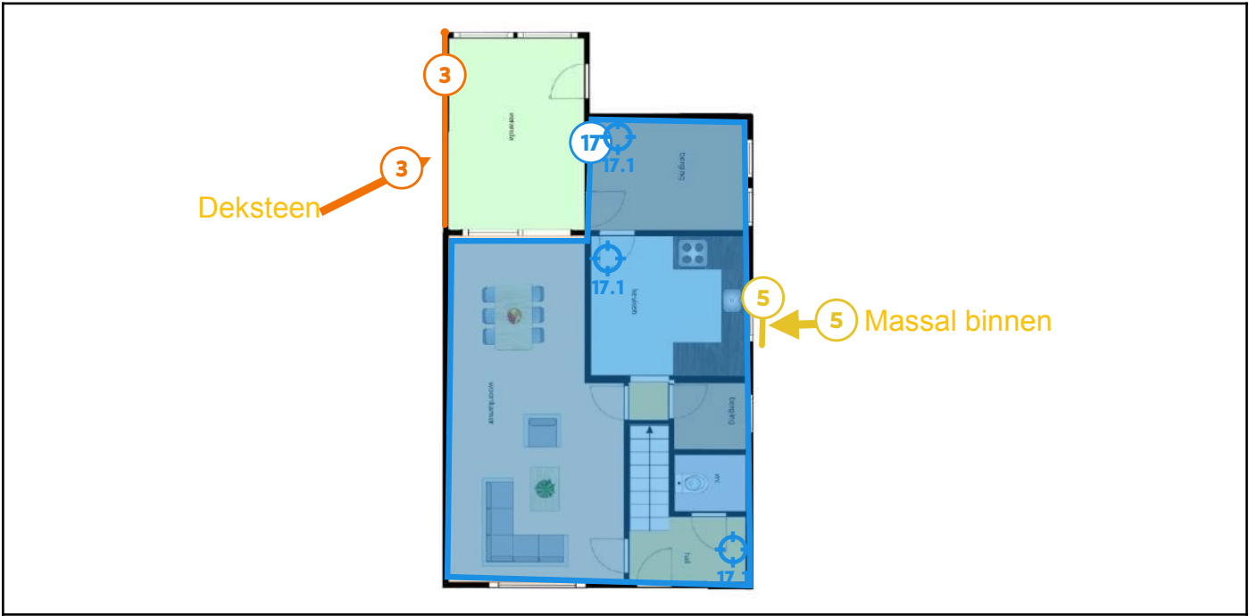
Legende van plan 1.2: Grondplan glvl kopie
