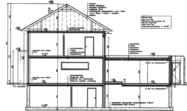
DOORSNEDEN A-B
