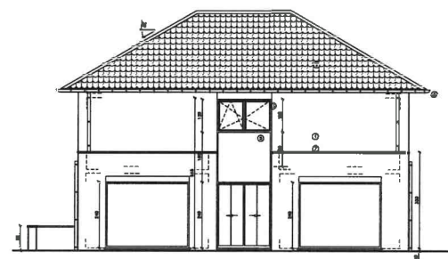
VOORGEVEL
