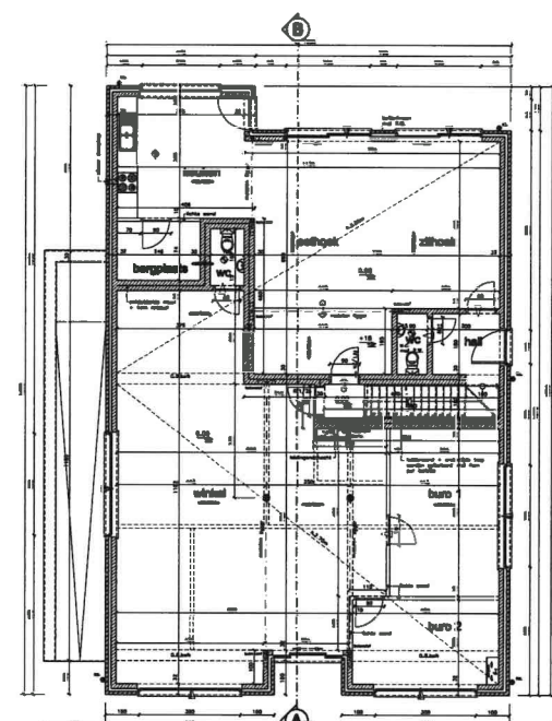
GELUKVLOERS
