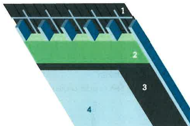
1. Onderdak | 2. Isolatie | 3. Dampscherm | 4. binnenaafwerking
