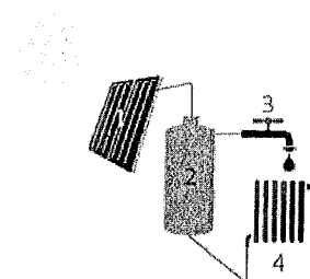
Een zonnecollector zet zonnepower om in warmte. Het opslagvat verwarmt het sanitair warm water met gratis zonnewarmte. De radiator verwarmt de ruimte met gratis zonnewarmte.
