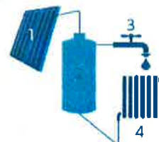
Zonnecollector (1) zonneboiler (2) en verwarming (3) en radiator (4)
