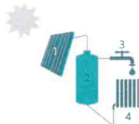
* Zonnecollector | 2. Opslagvat voor warm water | 3. Sanitair warm water | 4. Ruffte afgevoerd voor ruimteverwarming | 4. Ruffte afgevoerd voor ruimteverwarming
