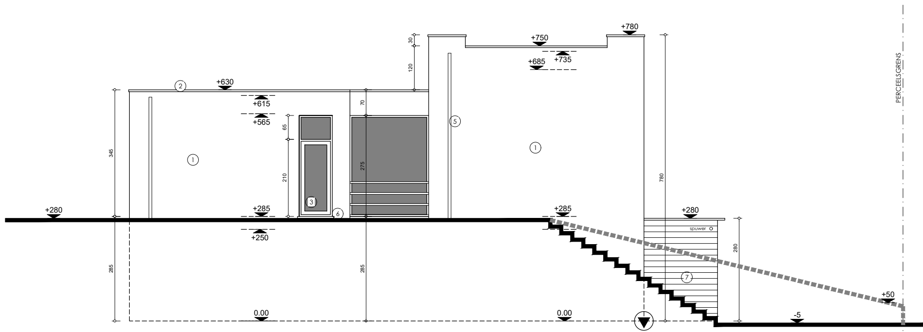
ZIJGEVEL LINKS
