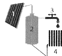
Fig. 2: Zonnecollectoren om warmte te produceren De zonnecollectoren zetten de energie van de zon om in warmte. Een zonneboilerinstallatie bestaat uit zonnecollectoren op het dak en een opslagvat voor warm water. Een zonneboiler verwarmt een deel van het sanitair warm water met gratis zonnewarmte. Als de installatie voldoende groot is, kan ze ook in een deel van uw behoefte voor ruimteverwarming voorzien. Hou er wel rekening mee dat een zonnecollector het hoogste rendement behaalt in de zomer. Het rendement in de winter ligt beduidend lager.
