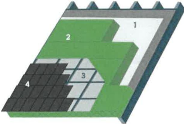
1. Dampschermbekleding | 2. Isolatatie | 3. Onderdak | 4. Dakbedekking
