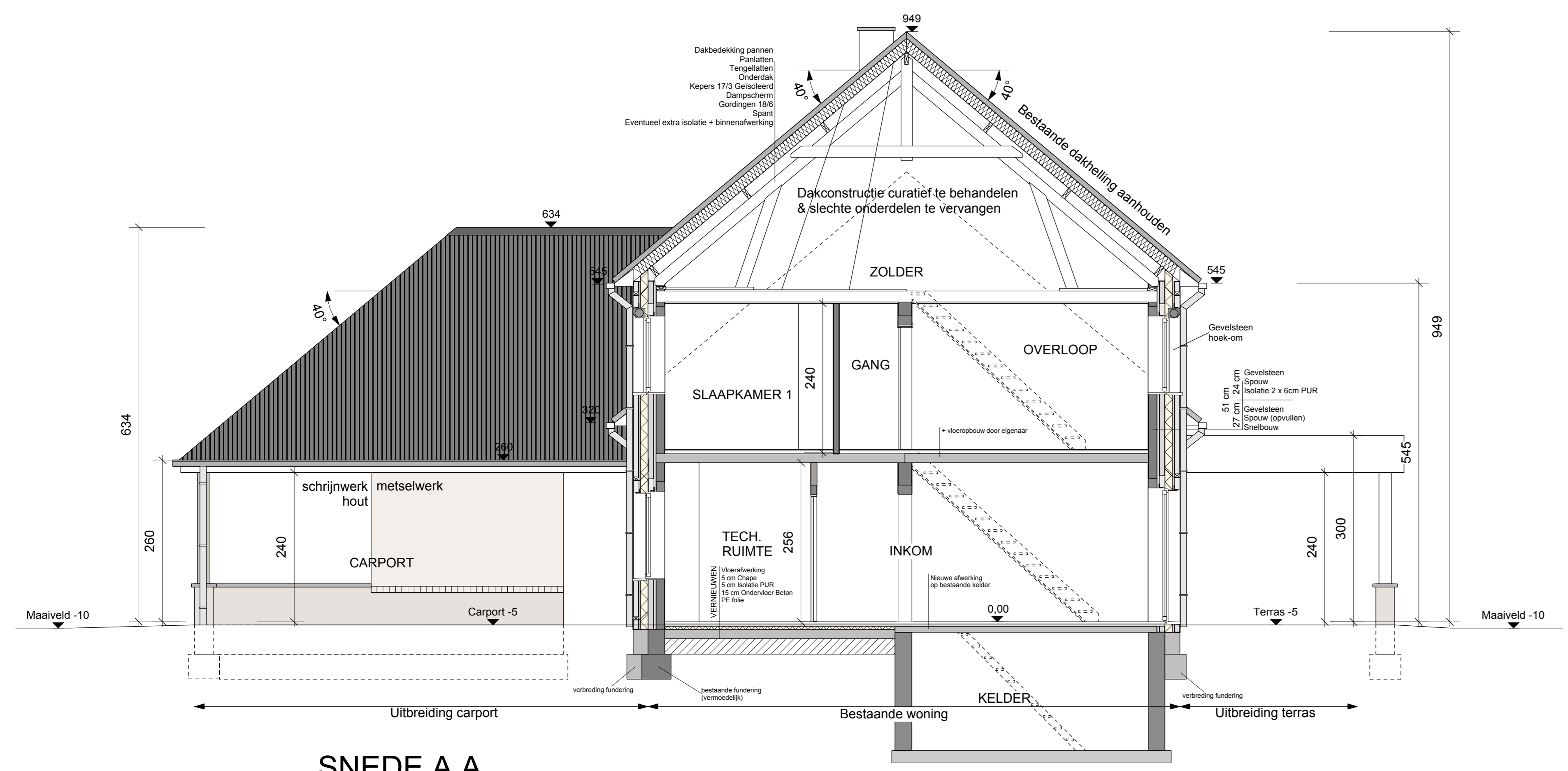
SNEDE A.A. NIEUWE TOESTAND SCHAAL 1/50
