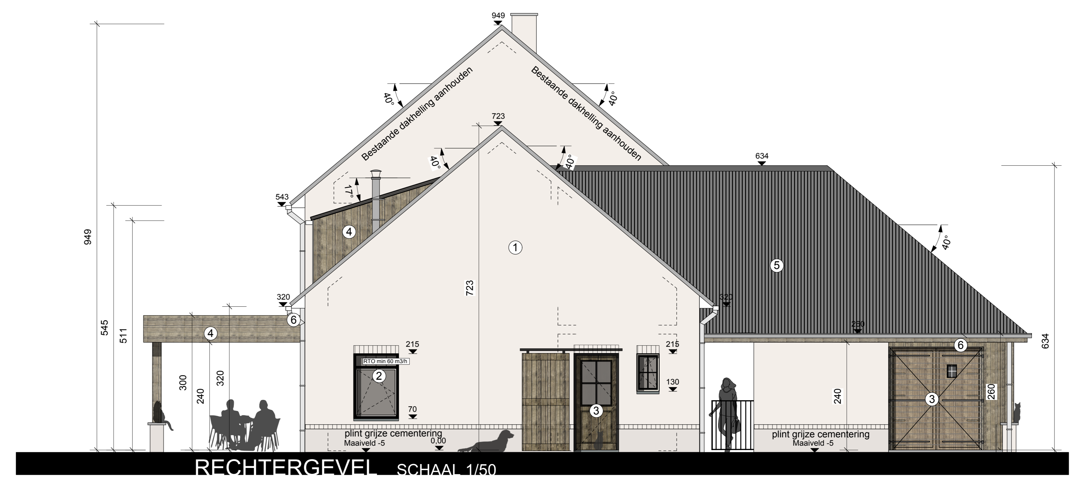
RECHTERGEVEL SCHAAL 1/50
