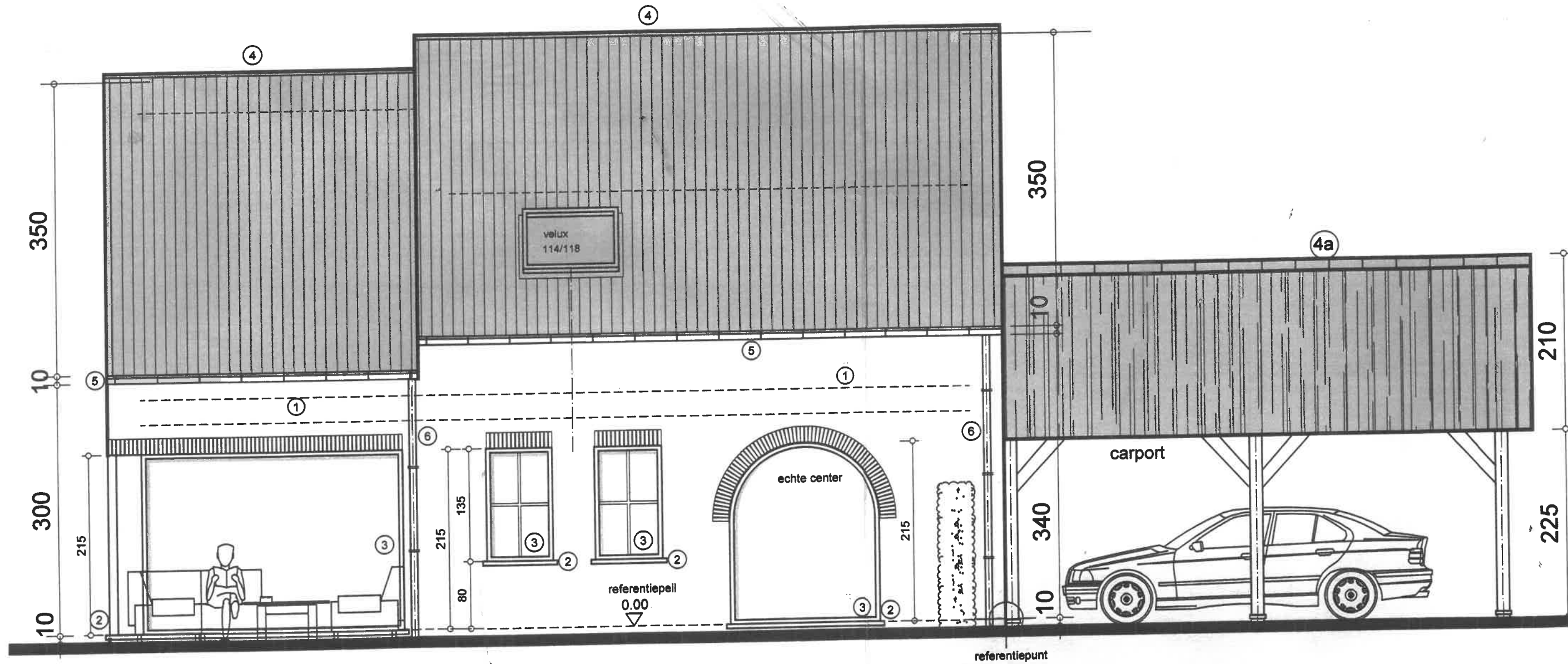
zijgevel links / 1:50
