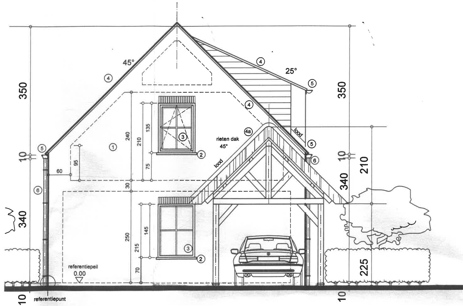
voorgevel / 1:50
