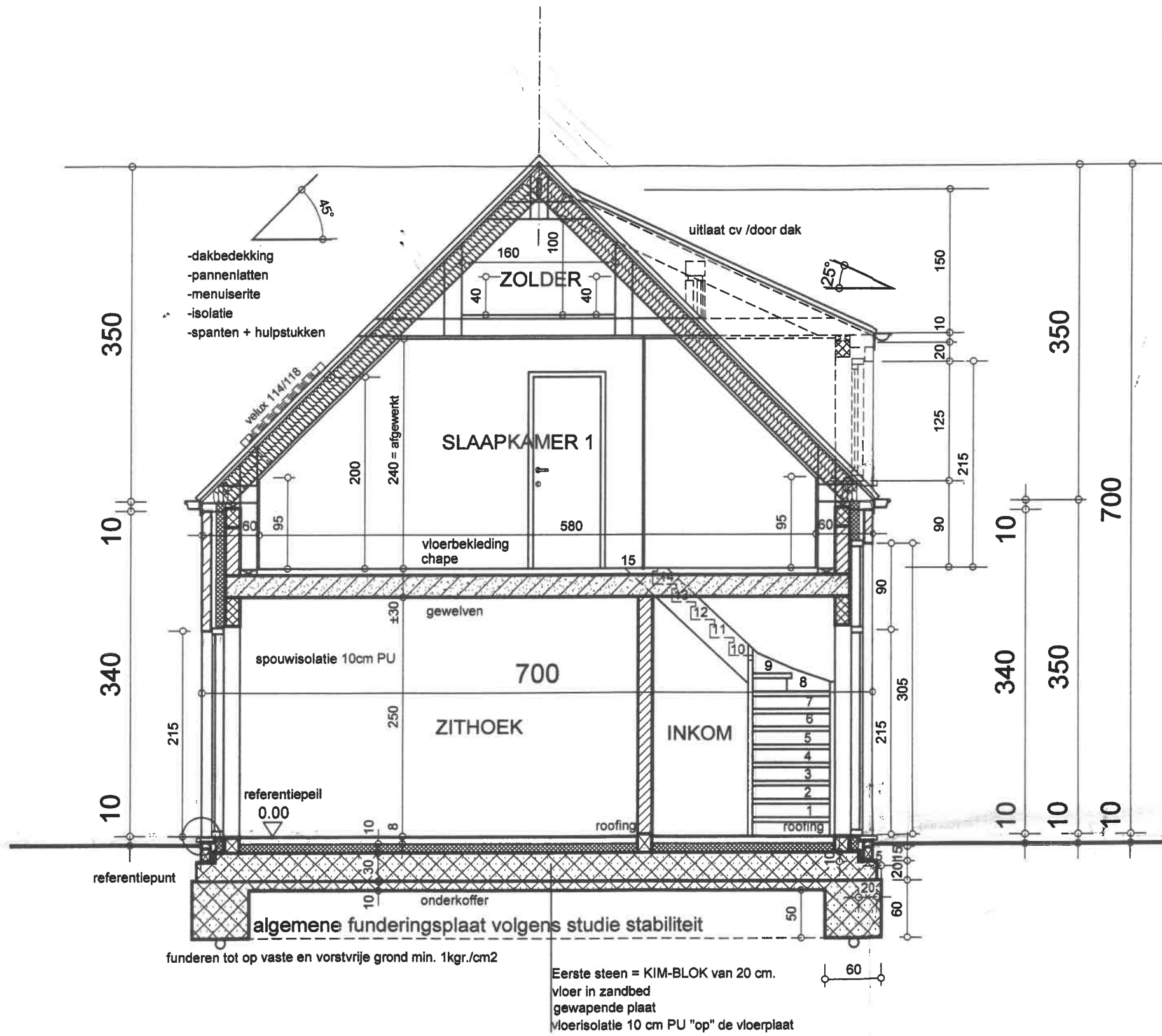
doorsnede aa / 1:50
