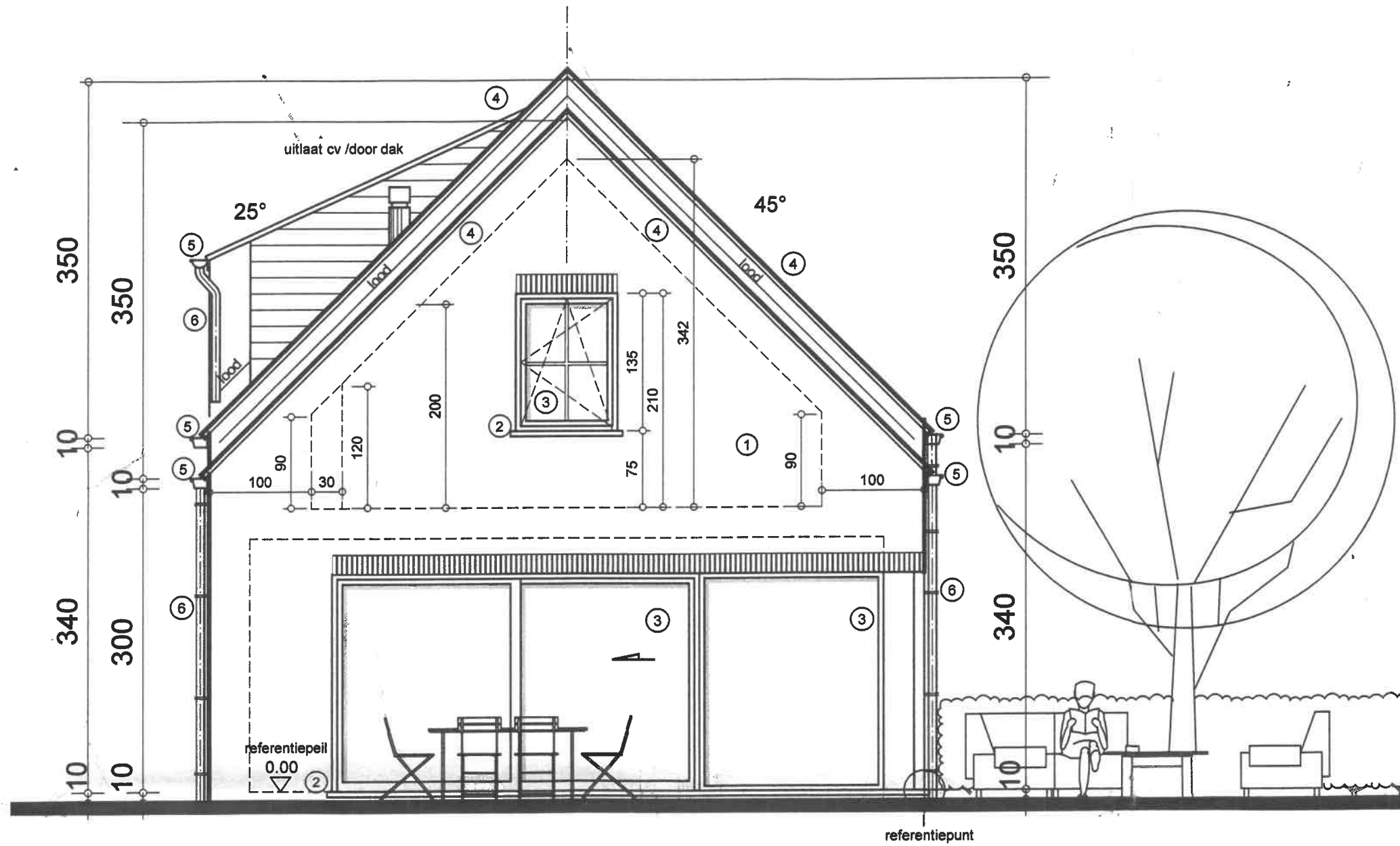
achtergevel / 1:50
