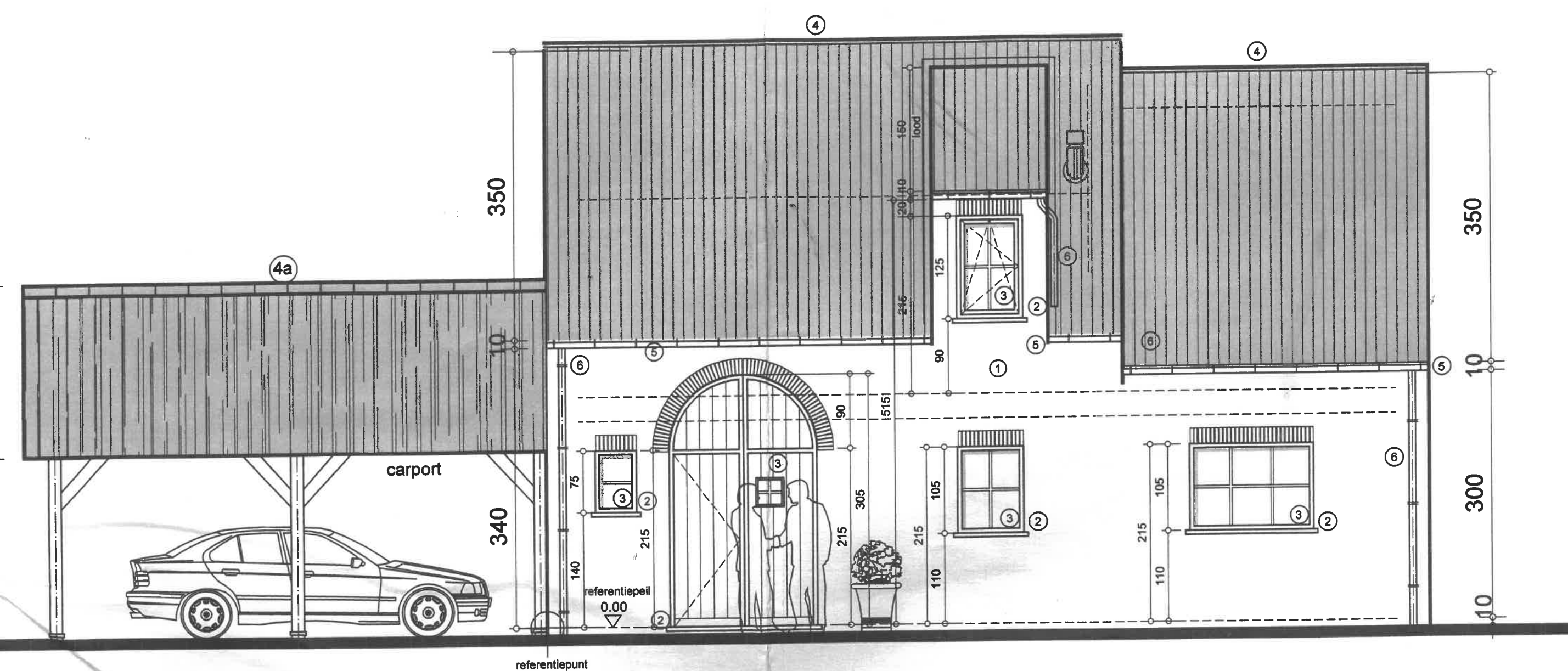
zijgevel rechts / 1:50
