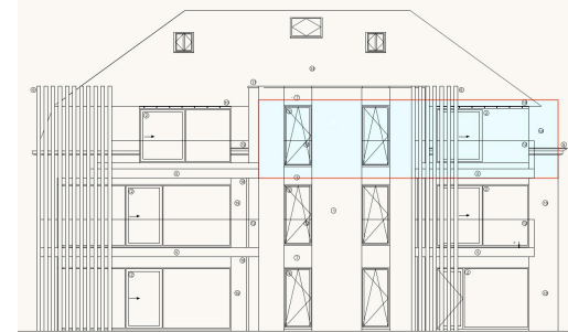
ACHTERGEVEL (NW)
