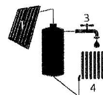
1. Zonnecollector | 2. Opslagvat zonneboiler | 3. Sanitair warm water | 4. Afgiftel element voor ruimteverwarming (opknop)
