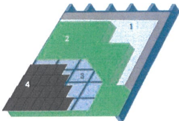
1. Dampscher姆 | 2. Isolatie | 3. Onderdak | 4. Dakbekleding
