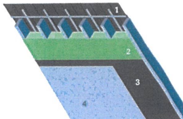
1. Onderdak | 2. Isolatie | 3. Dampscher姆 | 4. binnenafwerking
