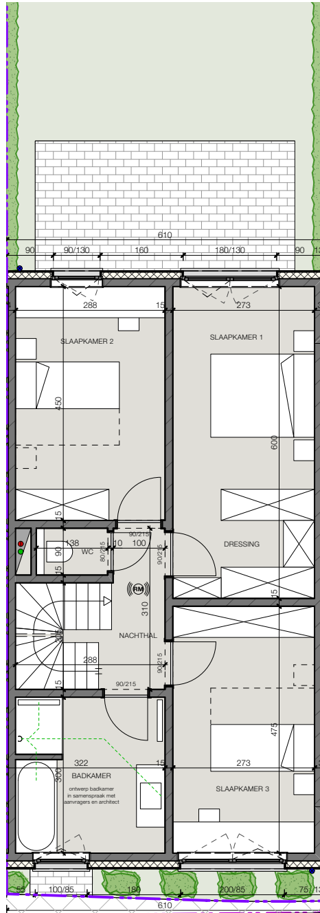
1° VERDIEPING WONING 3 Bruto: 70,15 m 2
