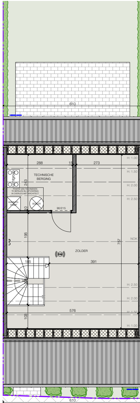
2° VERDIEPING WONING 3 Bruto: 53,11 m 2
