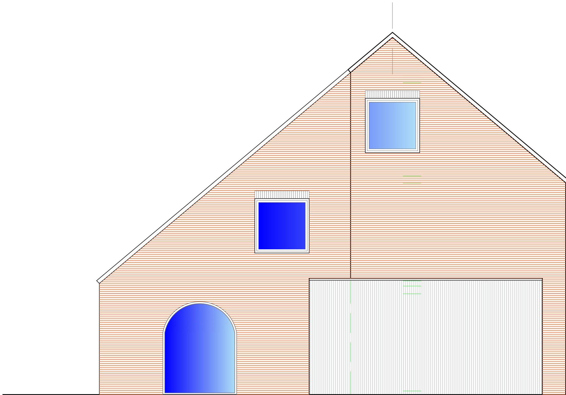
ZIJGEVEL LINKS
