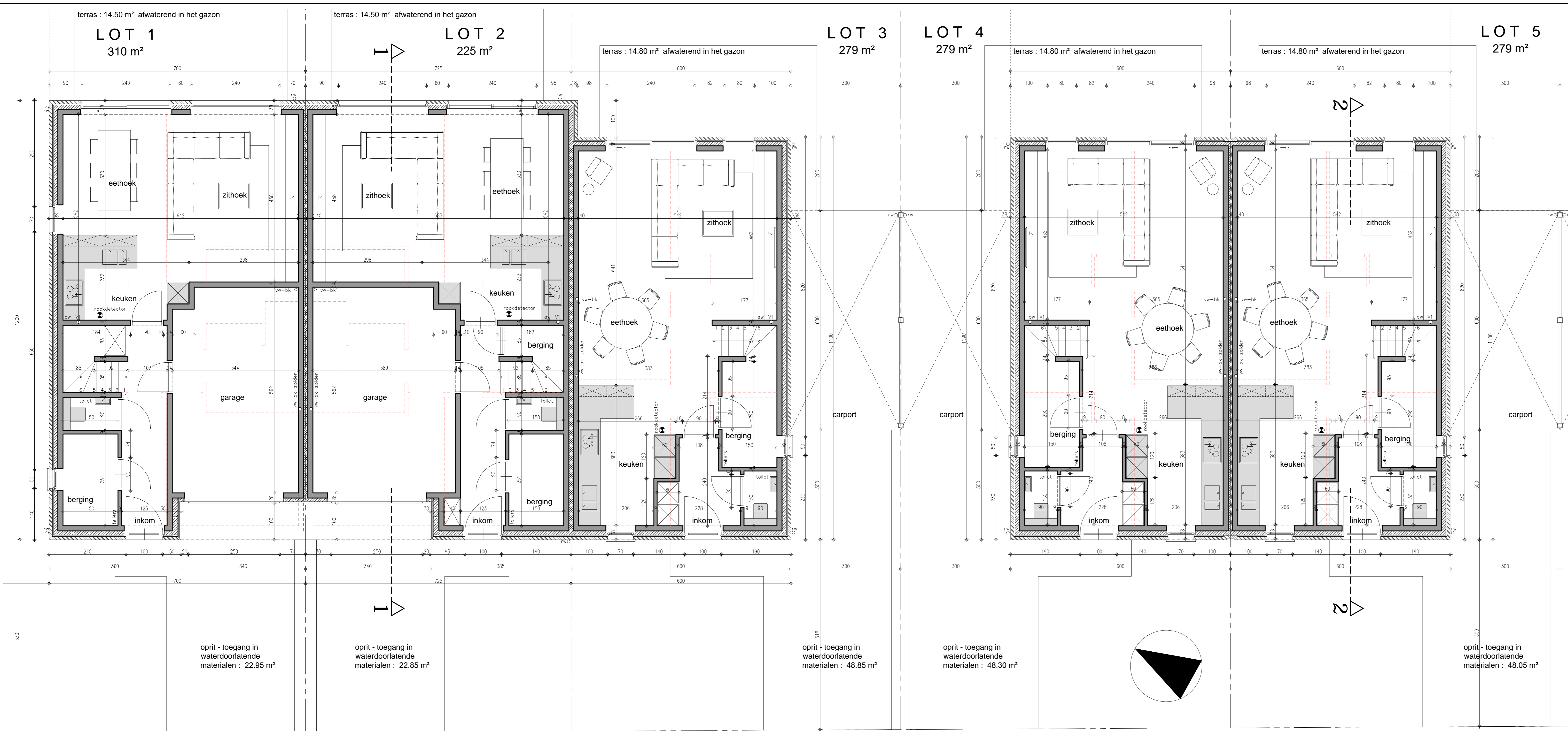
GELIJKVLOERS 1/50
